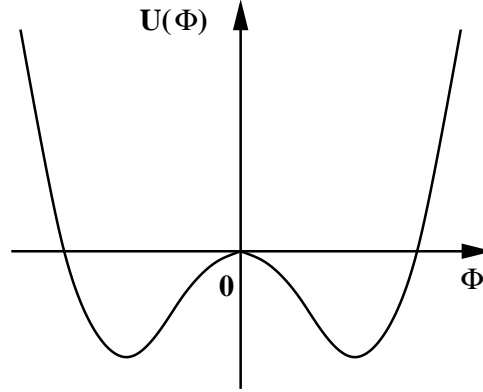
Abbildung 3: Das symmetrie-brechende Potential als Funktion der Variable \Phi .
