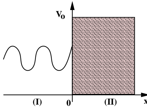
Abbildung 1: Schema zum Kleinschen Paradoxon.
