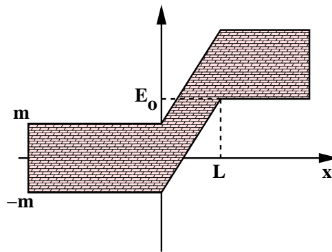
Abbildung 2: Schema zum Schwingermechanismus.
